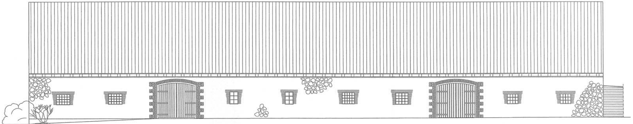
Vorderansicht
